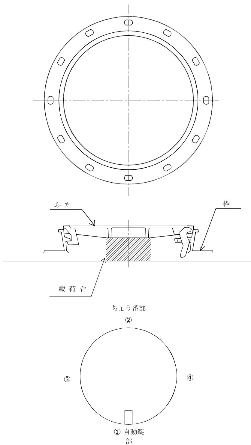
浮上しろ試験要領図
