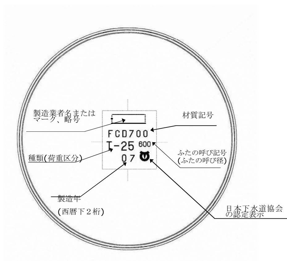
ふた裏面図
