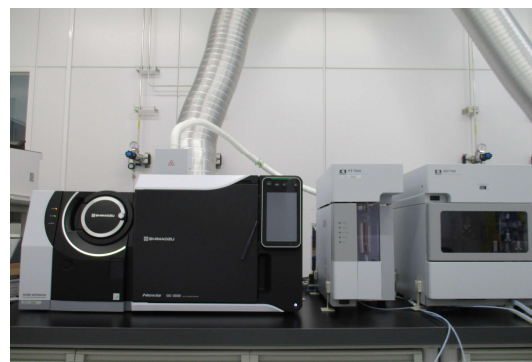
ページ・トラップガスクロマトグラフ質量分析装置 (島津製作所製GCMS-QP2020NX) (ジーエルサイエンス製PT7000)
