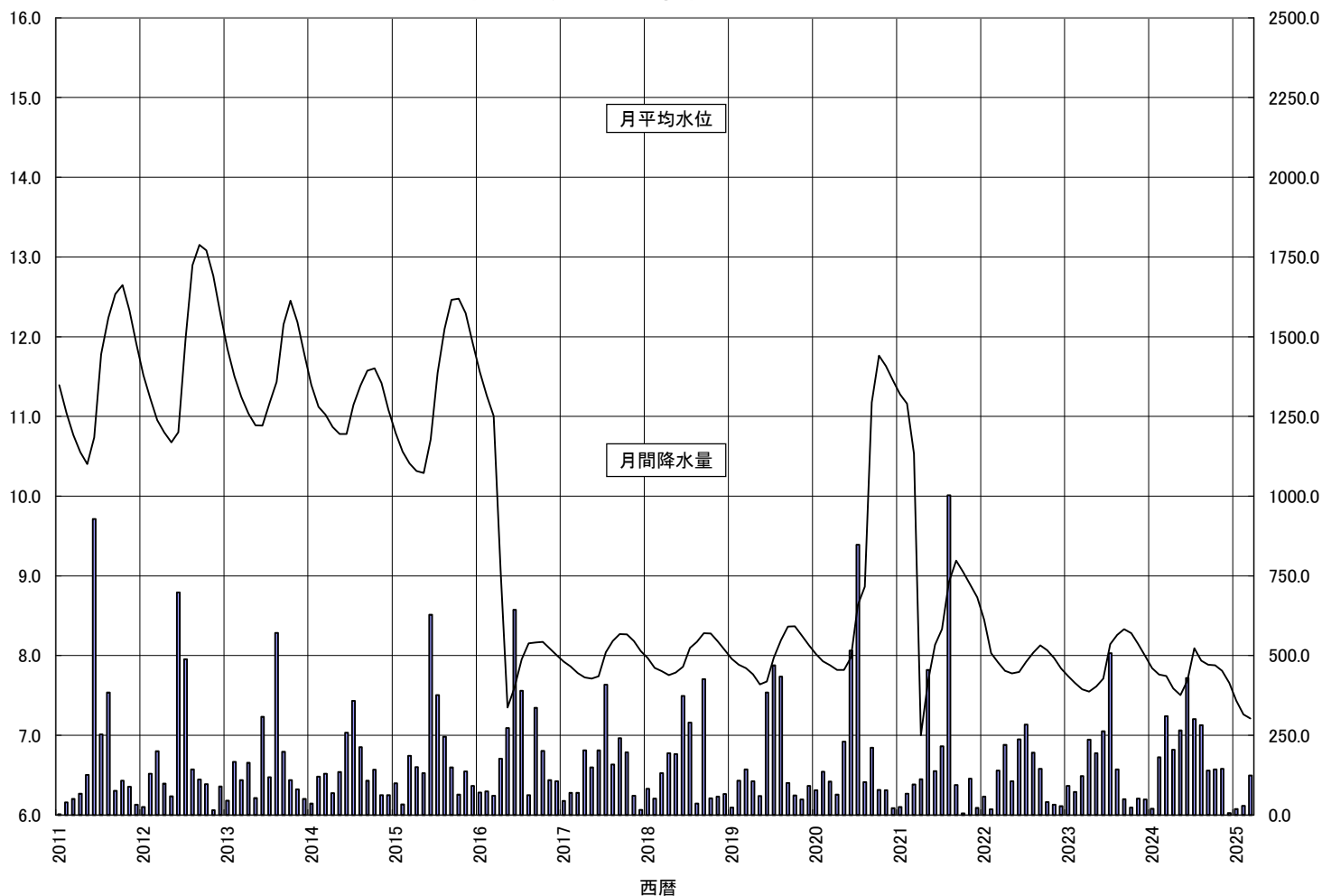
地下水水位標高データ
