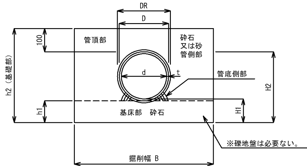
基礎寸法表
