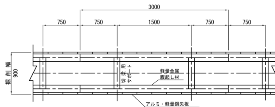
平面図
