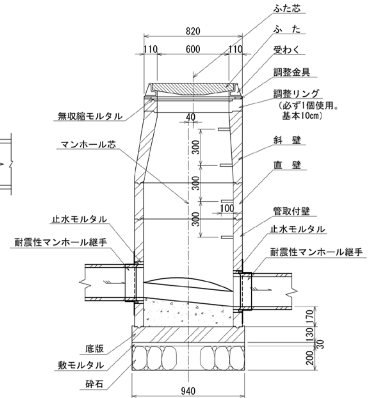
縦断面図
