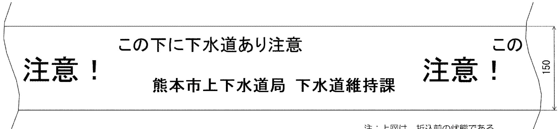
印刷表示図
