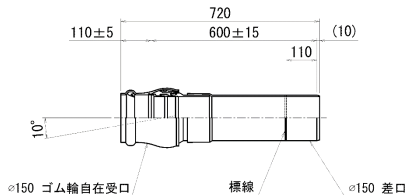
塩ビ管150mm 0°～10°
