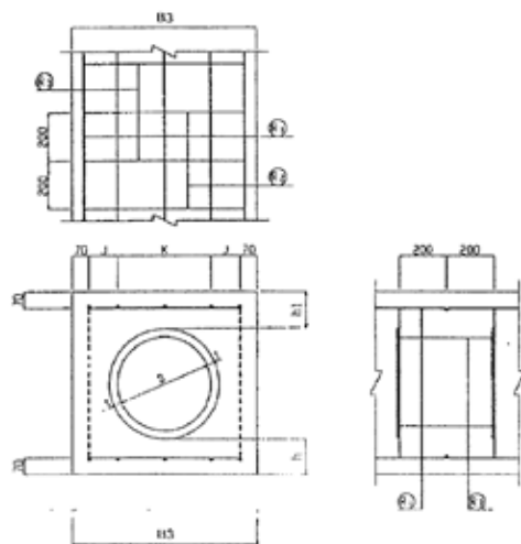
D 450～700mm
