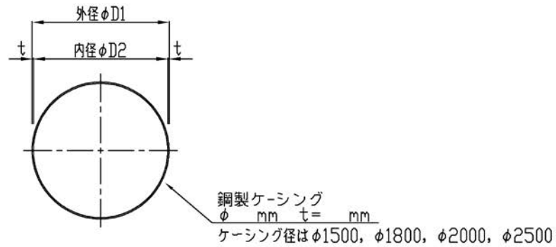
圧入掘削完了図
