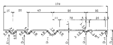
カラー詳細
