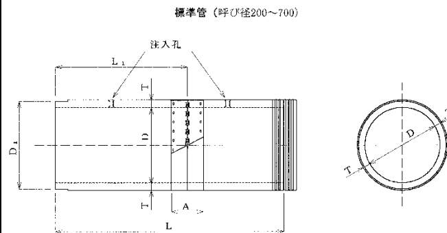
継手部詳細
