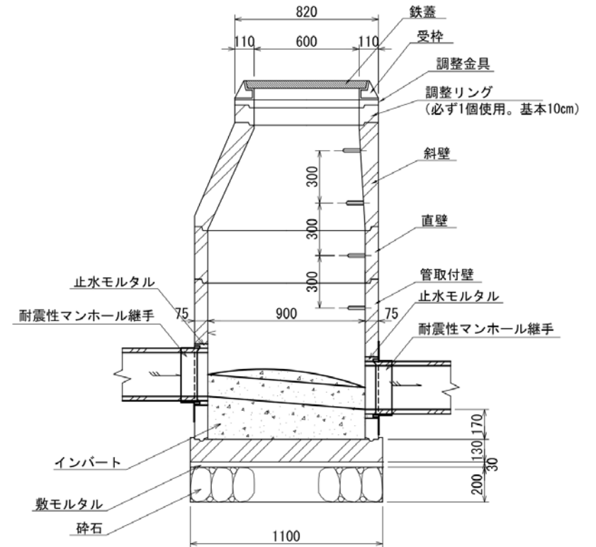
縦断面図
