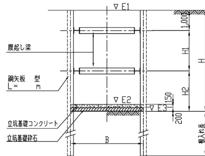
横断図
