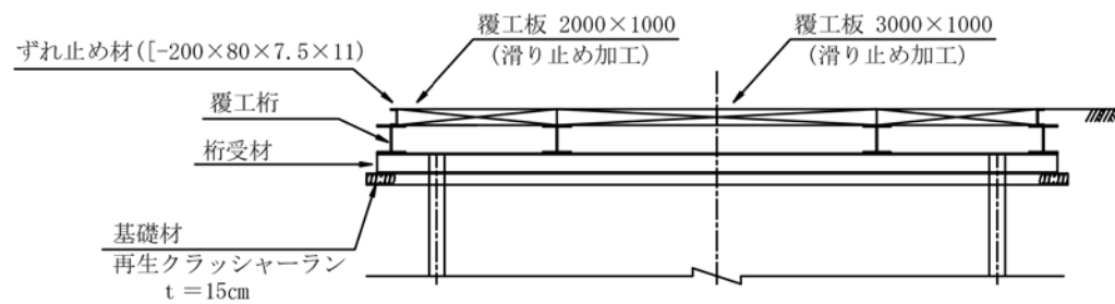
A-A 断面図
