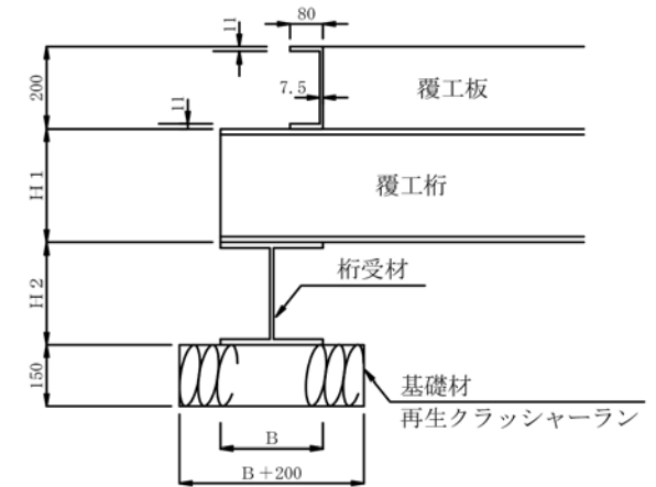
詳細図
