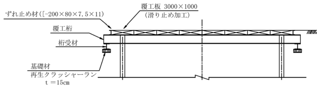
A-A 断面図
