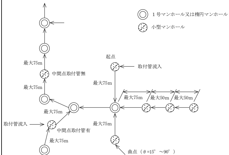
設置例
