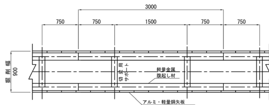
平面図
