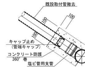
コンクリート防護断面図
