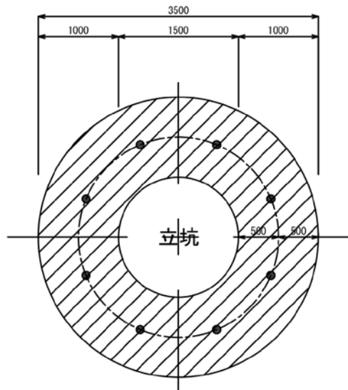
④改良深5.0m以下 側壁厚1.0m（坑口部なし） 平面図
