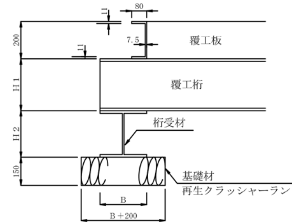
詳細図
