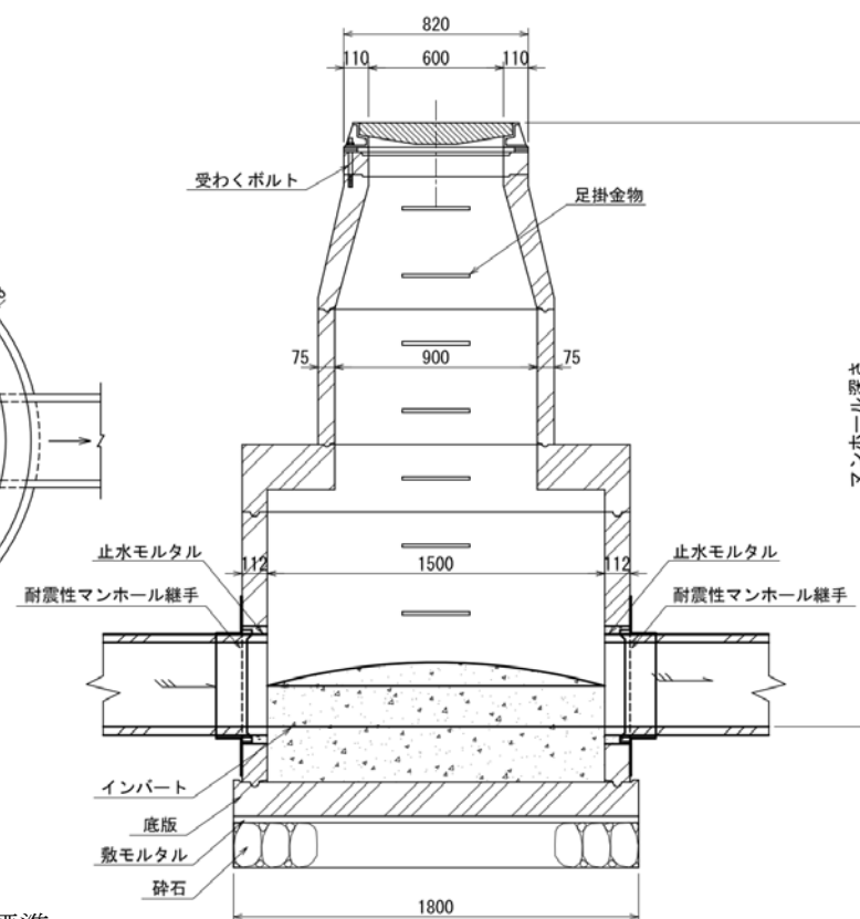
縦断面図
