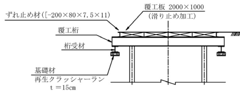
A-A 断面図
