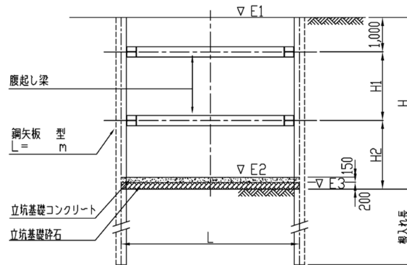
縦断図
