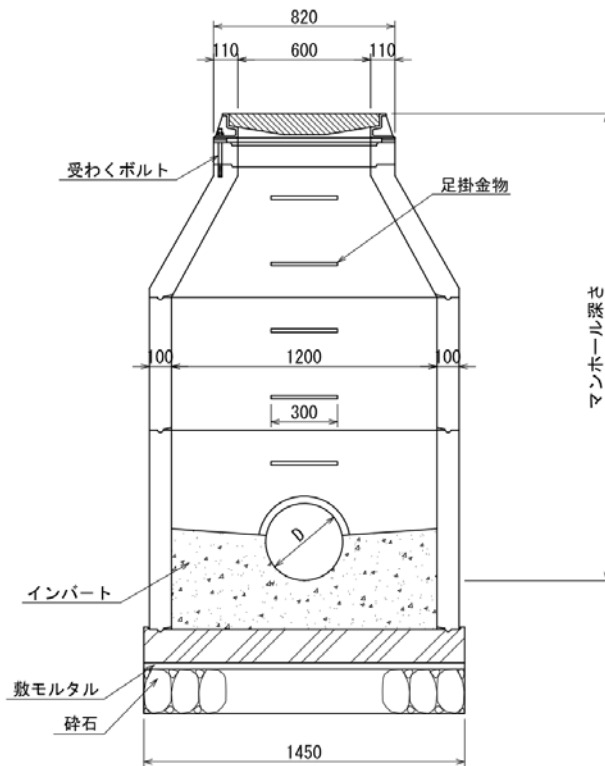
横断面図
