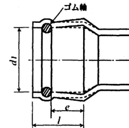
取付け管形
