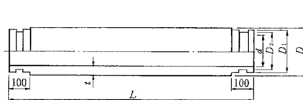
標準管
