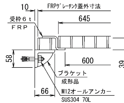
端部断面詳細図 （φ600開口部）
