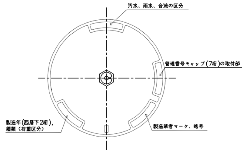
蓋表面図
