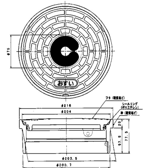
(硬質塩化ビニル製蓋)
