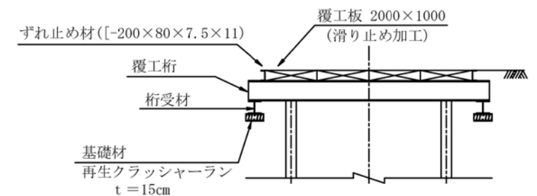
B-B 断面図
