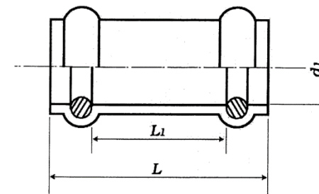
ゴム輪受口カラー (略号 WR)
