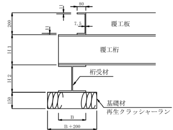
詳細図
