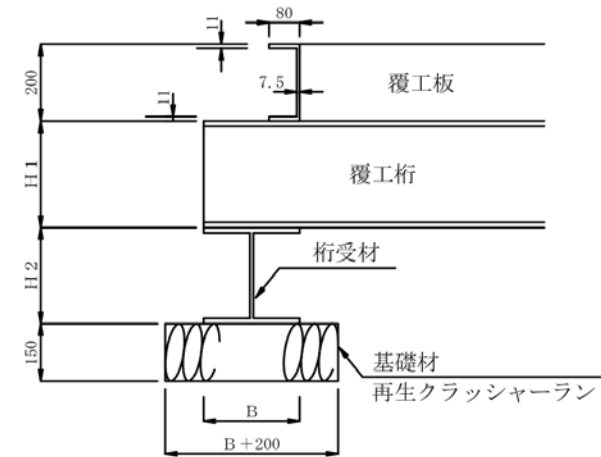
詳細図
