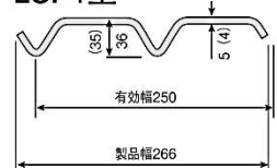
LSP1型
