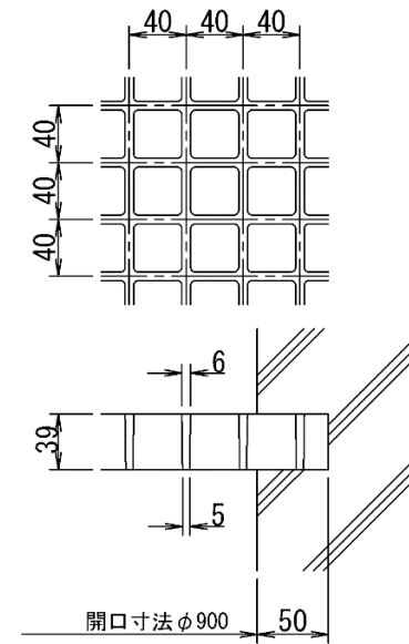
FRPグレーチング詳細図
