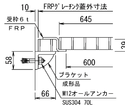
端部断面詳細図 （φ 600開口部）
