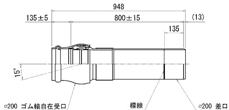
塩ビ管200mm 0°～15°
