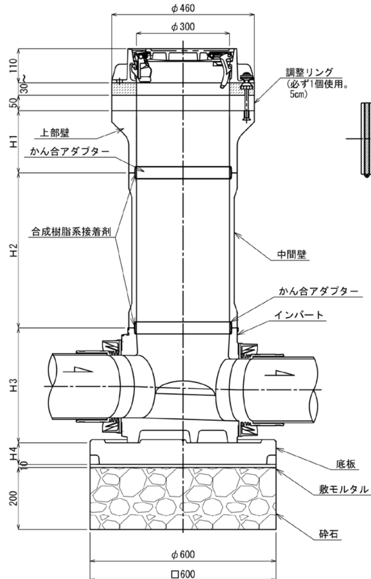
標準組立図
