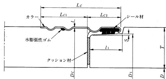
継手部詳細
