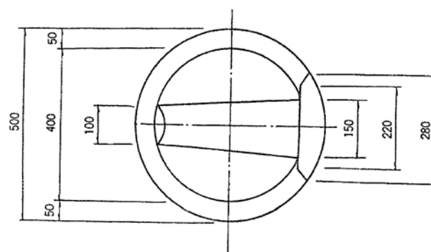
汚水枳 4 ブロック
