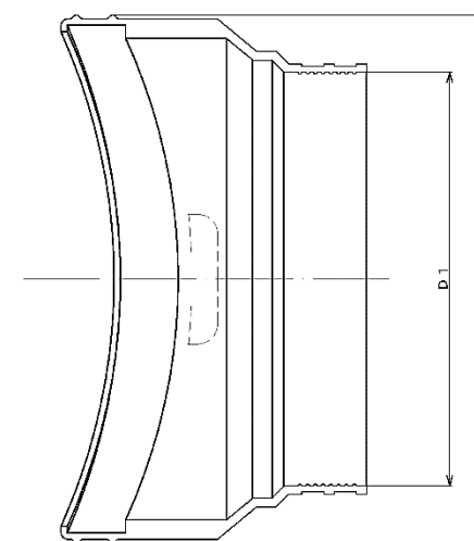
参考図 φ 400 まで
