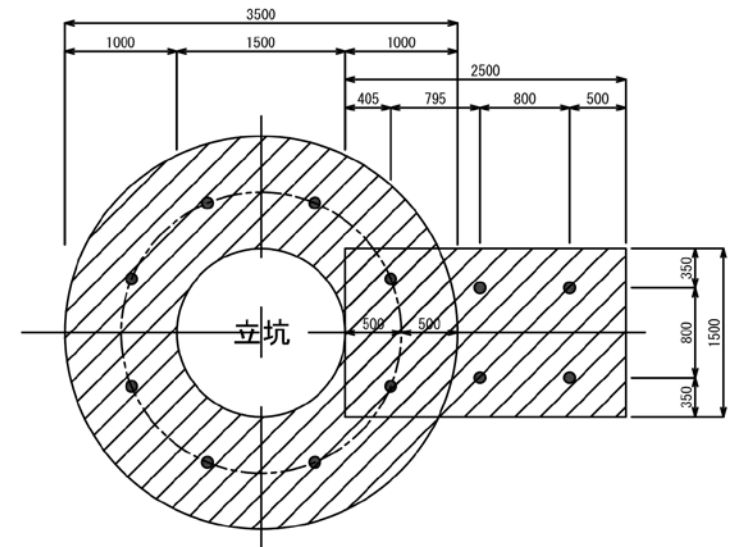
⑥改良深5.0m以下 側壁厚1.0m（坑口部1.5m×2.5m） 平面図
