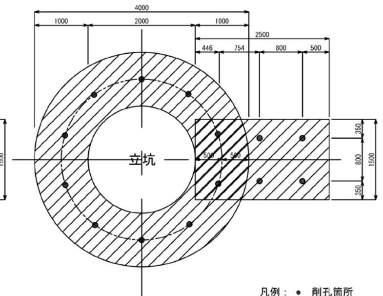
⑫改良深5.0m以下 側壁厚1.0m（坑口部1.5m×2.5m） 平面図
