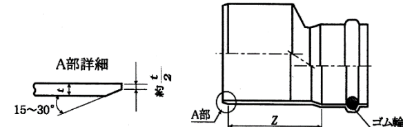
硬質塩化ビニル製小型マンホール用本管異径継手 (略号 IHR)
