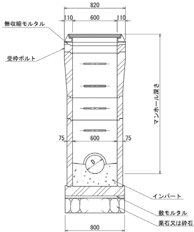
横断面図
