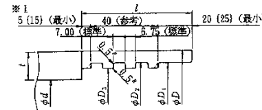
接続部参考図
