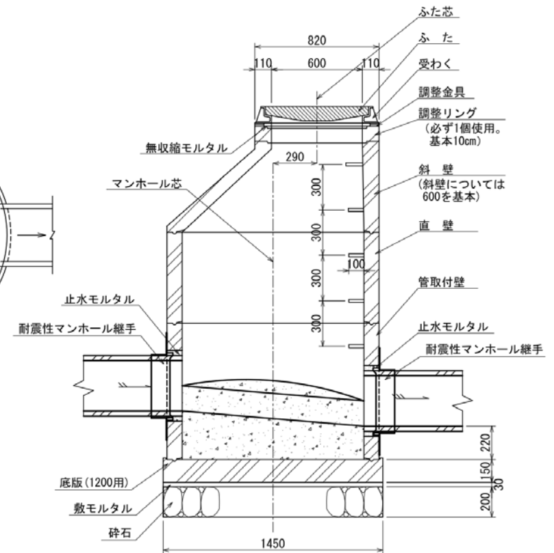
縦断面図
