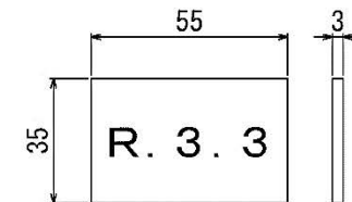
完成プレート 仕様（参考）
