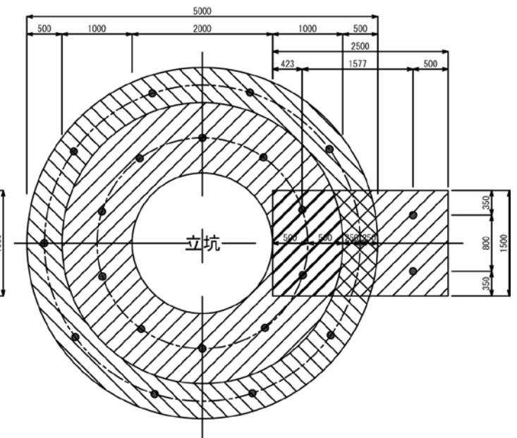
平面図
