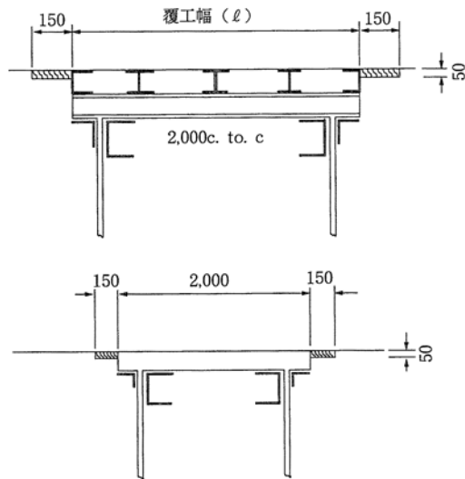
覆工板設置工図
