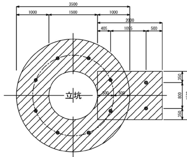
⑤改良深5.0m以下 側壁厚1.0m（坑口部1.5m×2.0m） 平面図
