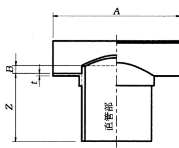
強化プラスチック複合管用副管 90 度支管 (略号 KS)
