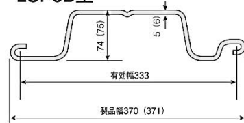
LSP3B型
