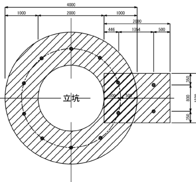
⑪改良深5.0m以下 側壁厚1.0m（坑口部1.5m×2.0m） 平面図
