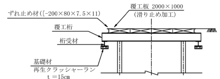
B-B 断面図
