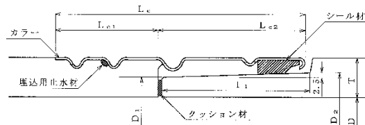
カラー詳細
