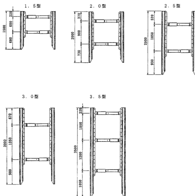
スライドレール方式
