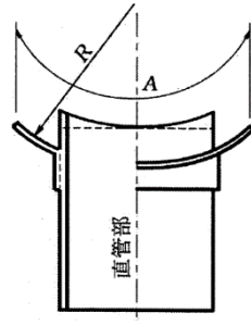
強化プラスチック複合管用副管 90 度支管 (略号 KS)
