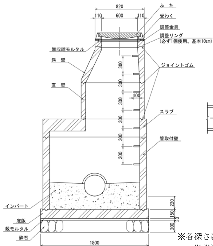
横断面図
