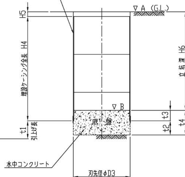
鋼製ケーシング \phi mm t = mm
