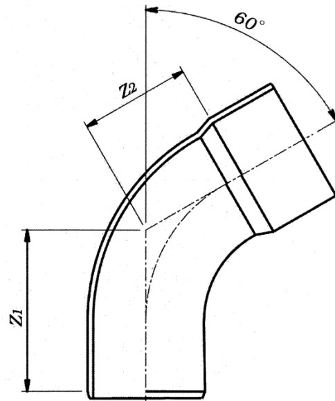
60 度曲管 接着受口 (略号 60ST)
