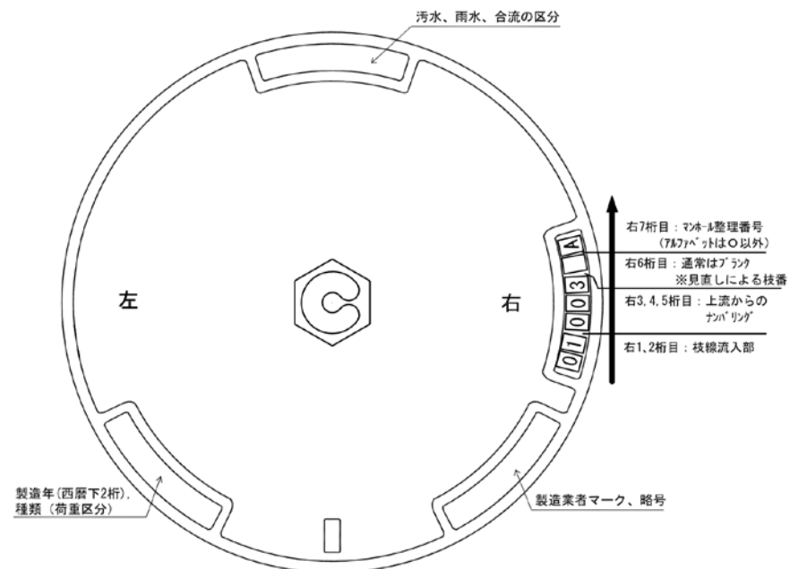
ふた 表面 図
