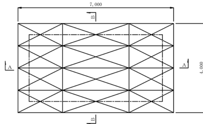
平面図
