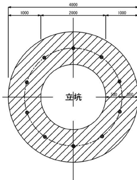
⑩改良深5.0m以下 側壁厚1.0m（坑口部なし） 平面図
