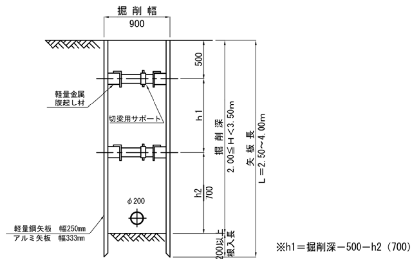
断面図 タイプ②
