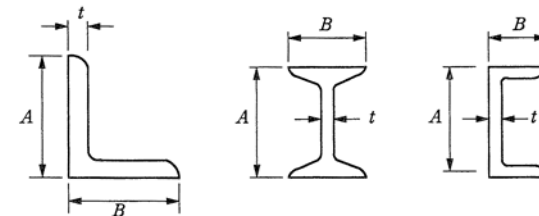
鋼材断面形状
