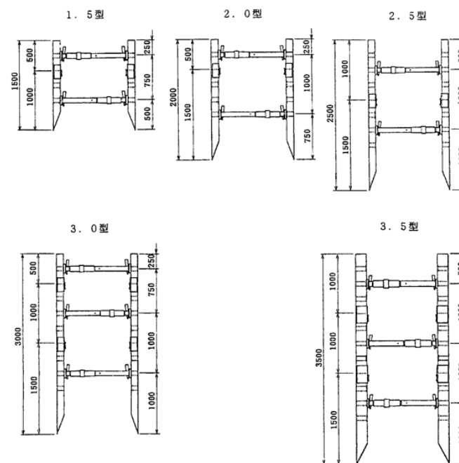
縦梁プレート方式
