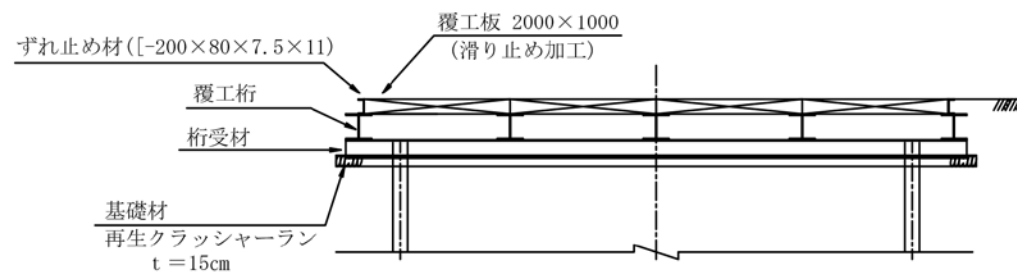
A-A 断面図
