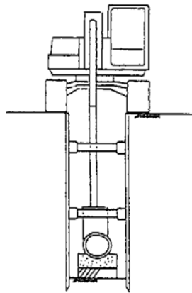
バックホウ
