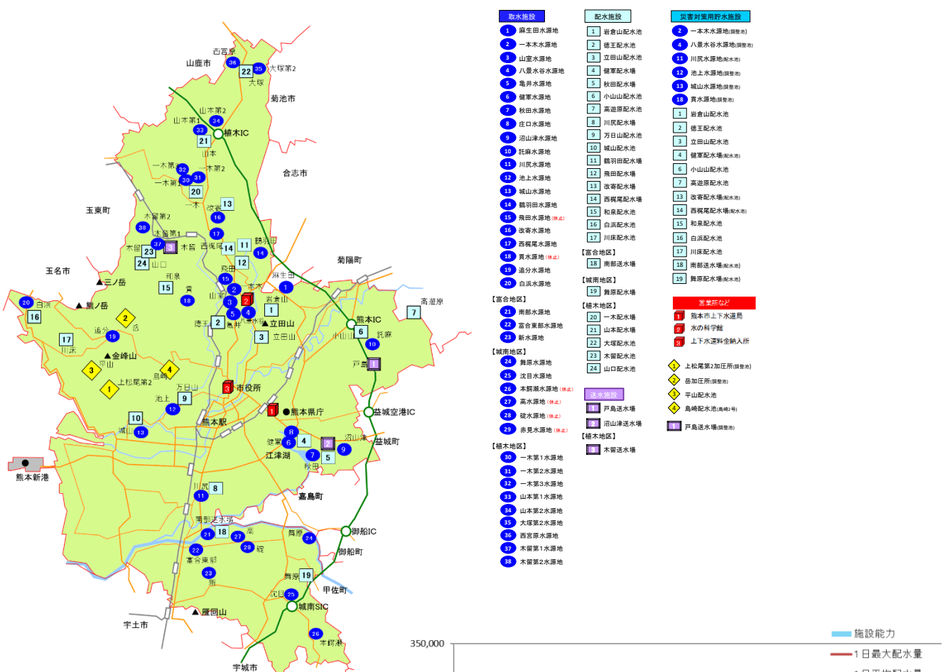
図 2-1-3 水道施設位置図
