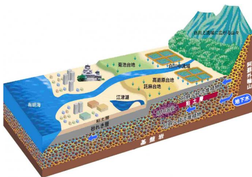
図 3-2-2-1 熊本地域の地層
