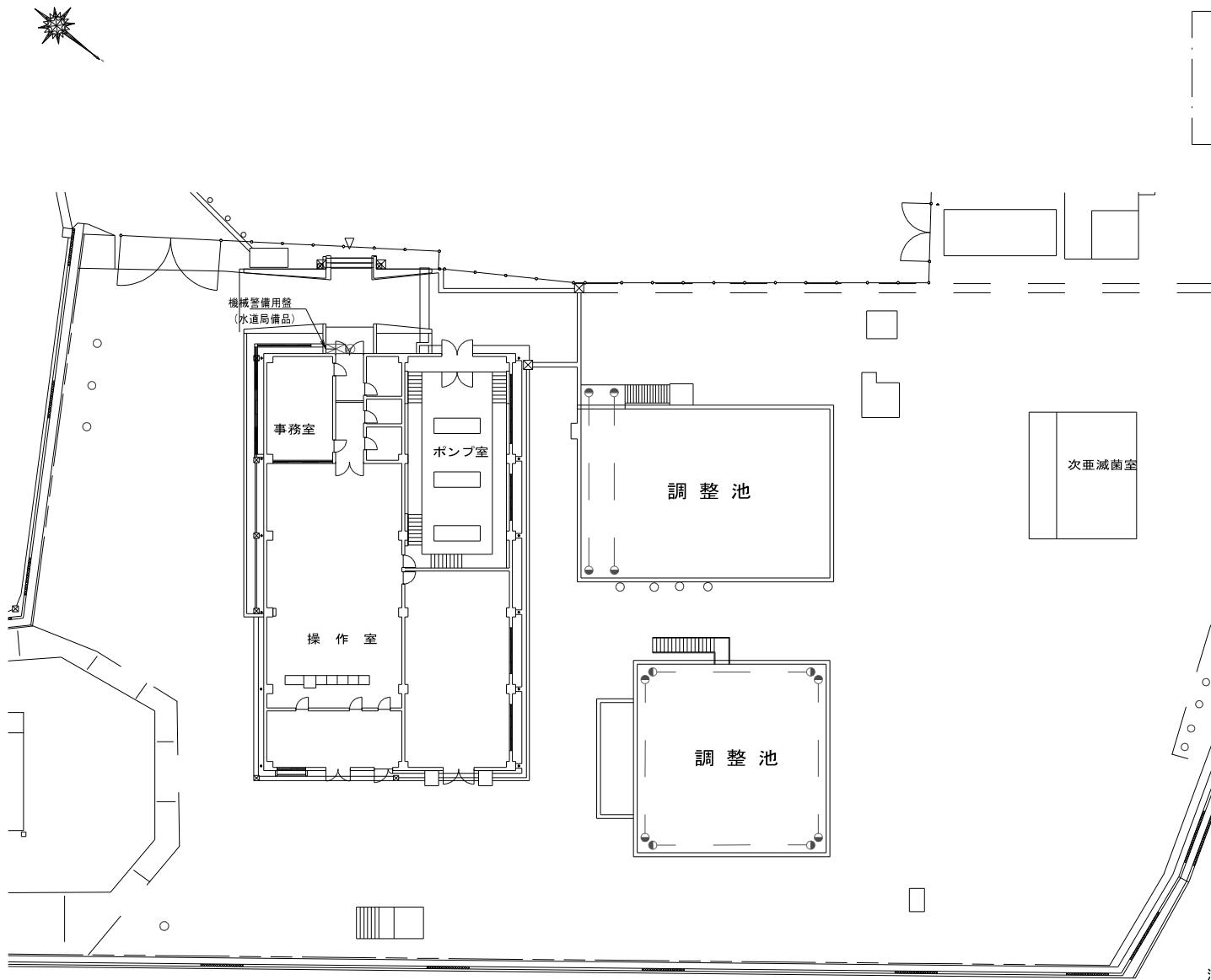
池上水源地構内平面図 (S=1/300)
