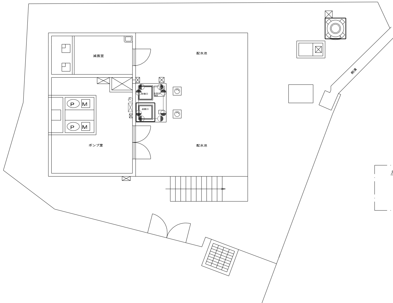
沈目水源地平面図 (S=1/150)
