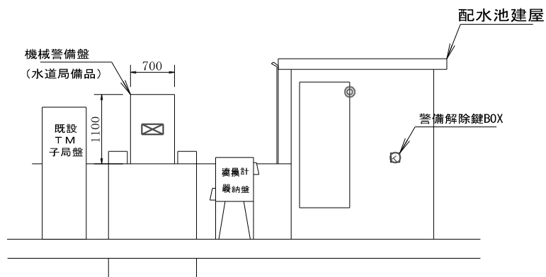
城山第2配水池建屋部立面図（S＝1／60） （機械警備機器設置参考図）
