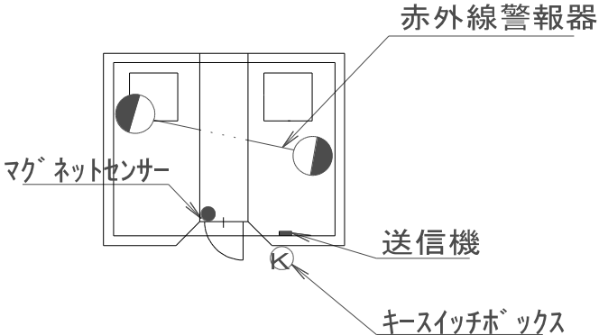
A部拡大図 (S=1/100)
