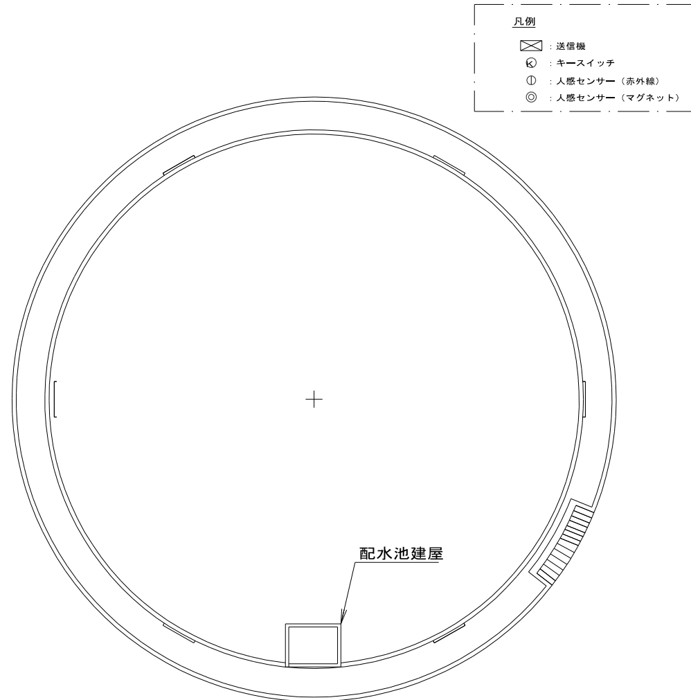
城山第2配水池構内平面図(S=1/150)
