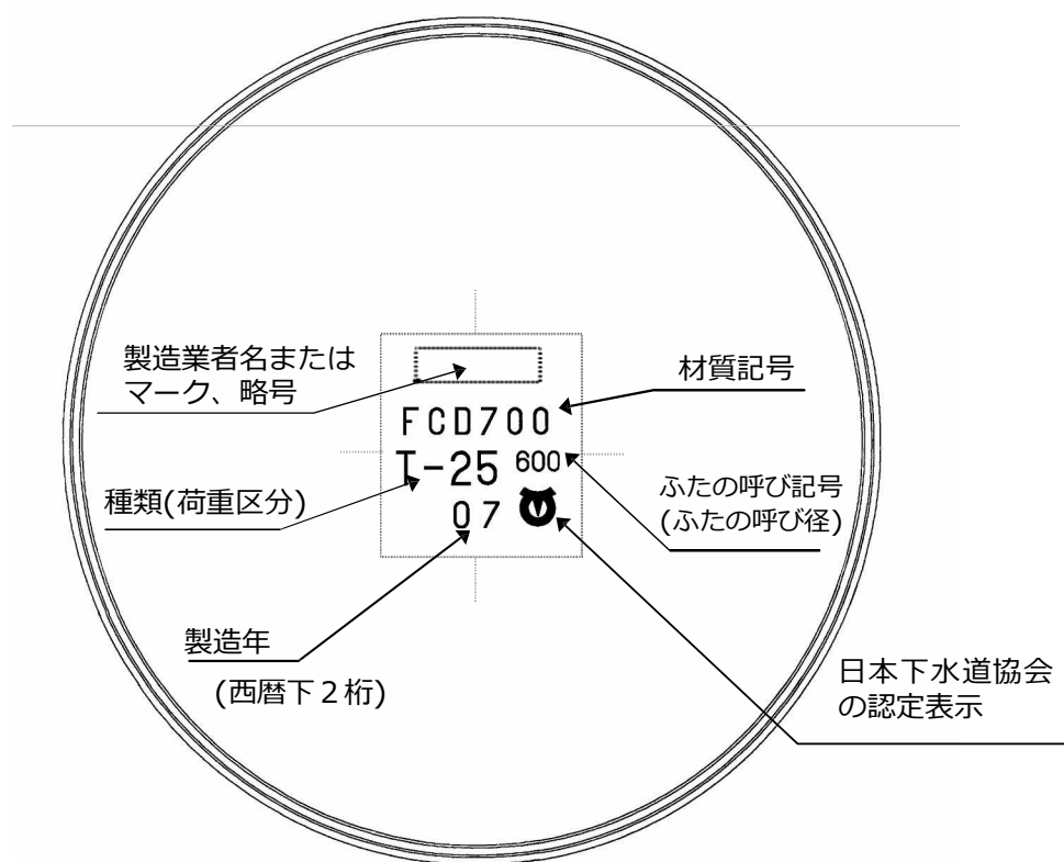
ふた裏面図
