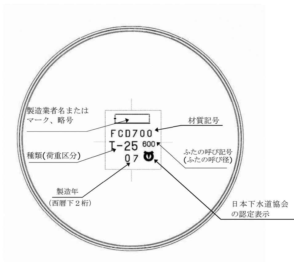
ふた裏面図
